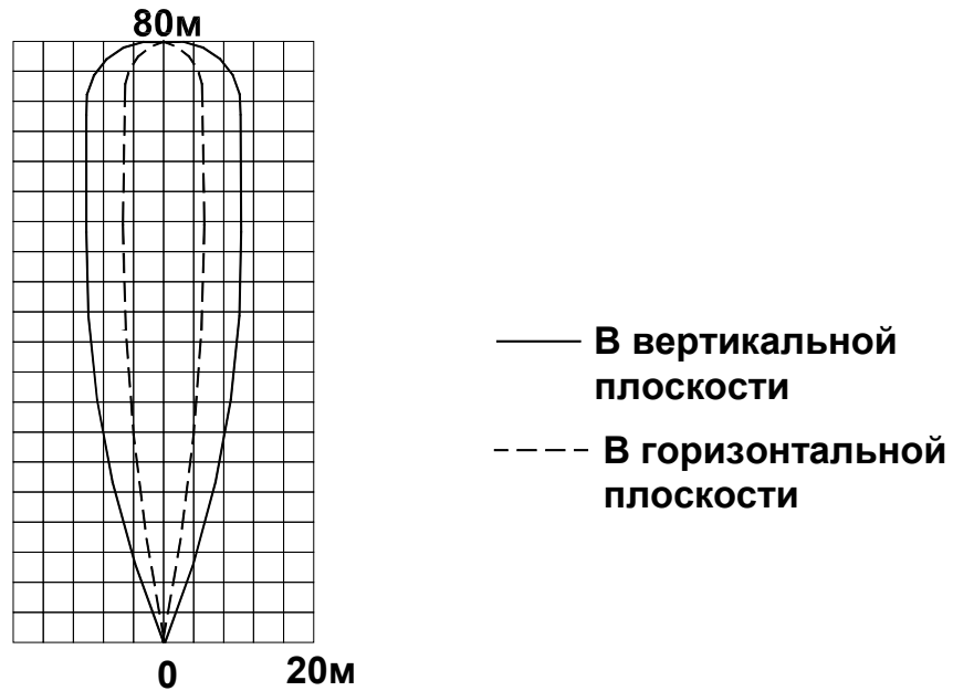
Примерная форма зоны обнаружения извещателя АГАТ-СП5У/2 при максимальной дальности
